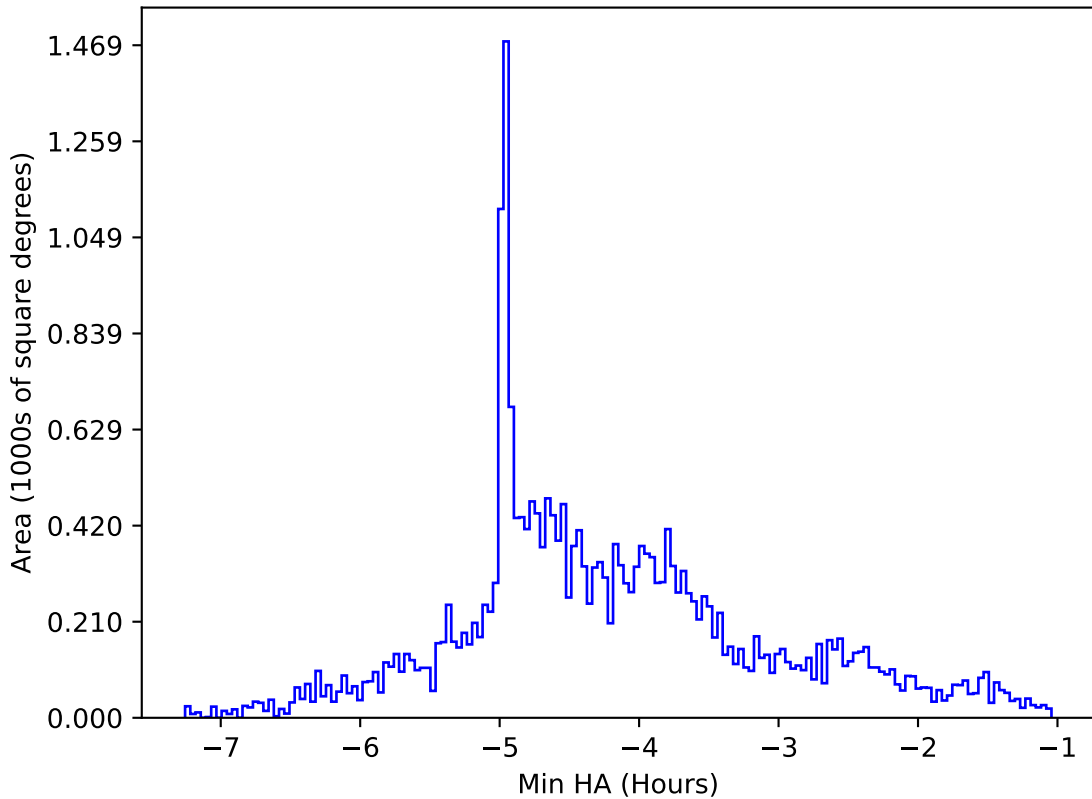
too_100_4v3.4_10yrs All sky g band: Min HA
