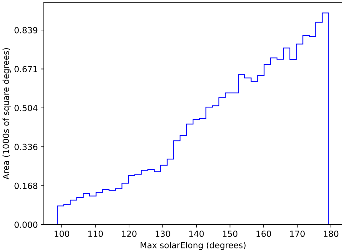
too_100_4v3.4_10yrs WFD y band: Max solarElong
