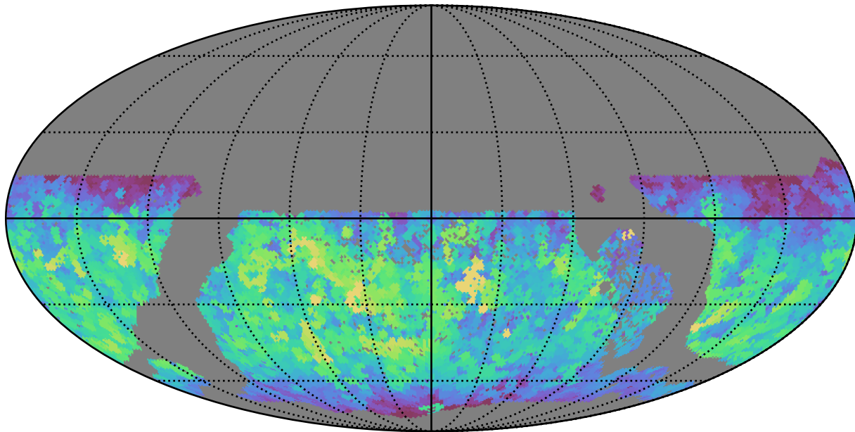
too_100_4v3.4_10yrs WFD y band: Max saturation_mag
