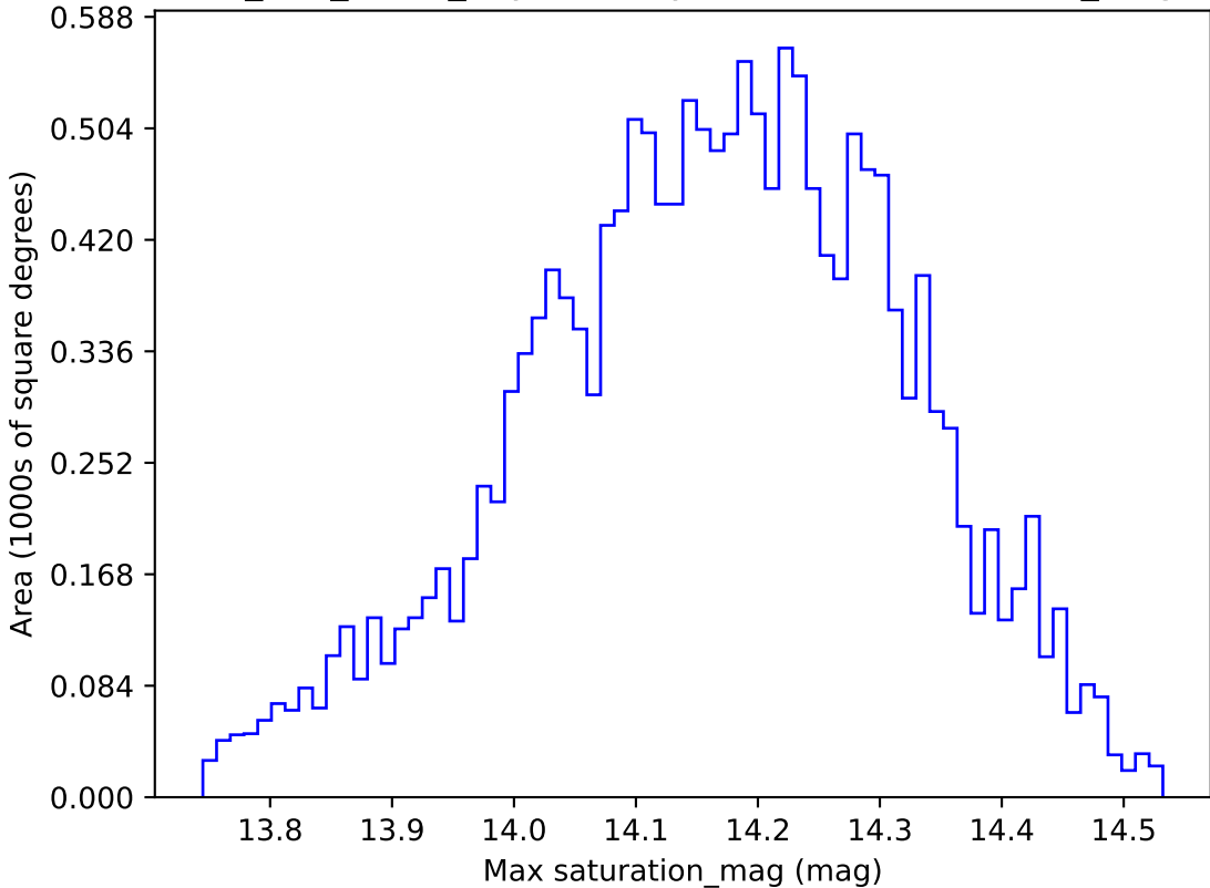
too_100_4v3.4_10yrs WFD y band: Max saturation_mag
