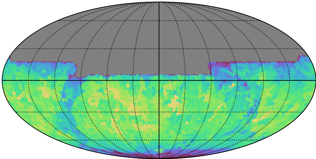
too_100_4v3.4_10yrs All sky y band: Max saturation_mag
