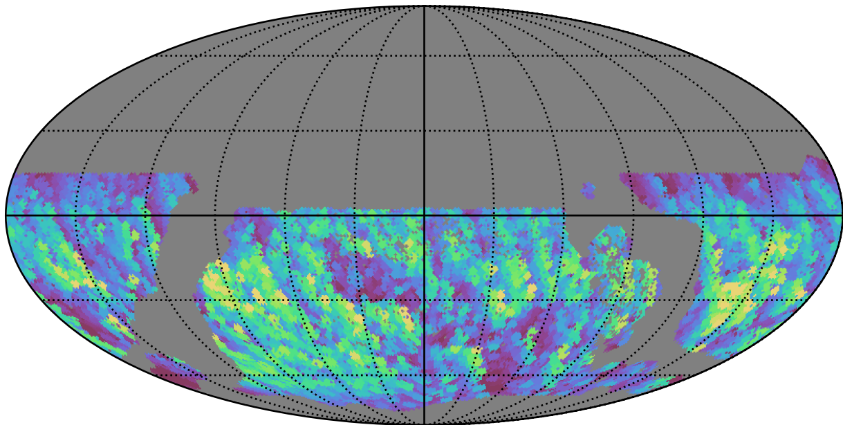
too_100_4v3.4_10yrs WFD y band: Max normairmass
