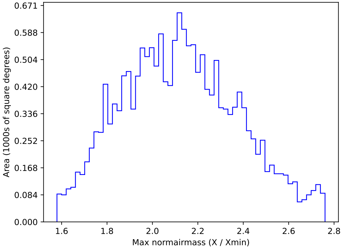
too_100_4v3.4_10yrs WFD y band: Max normairmass
