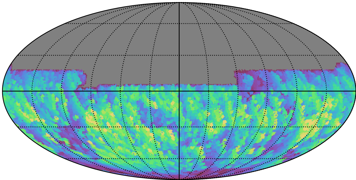
too_100_4v3.4_10yrs All sky y band: Max normairmass
