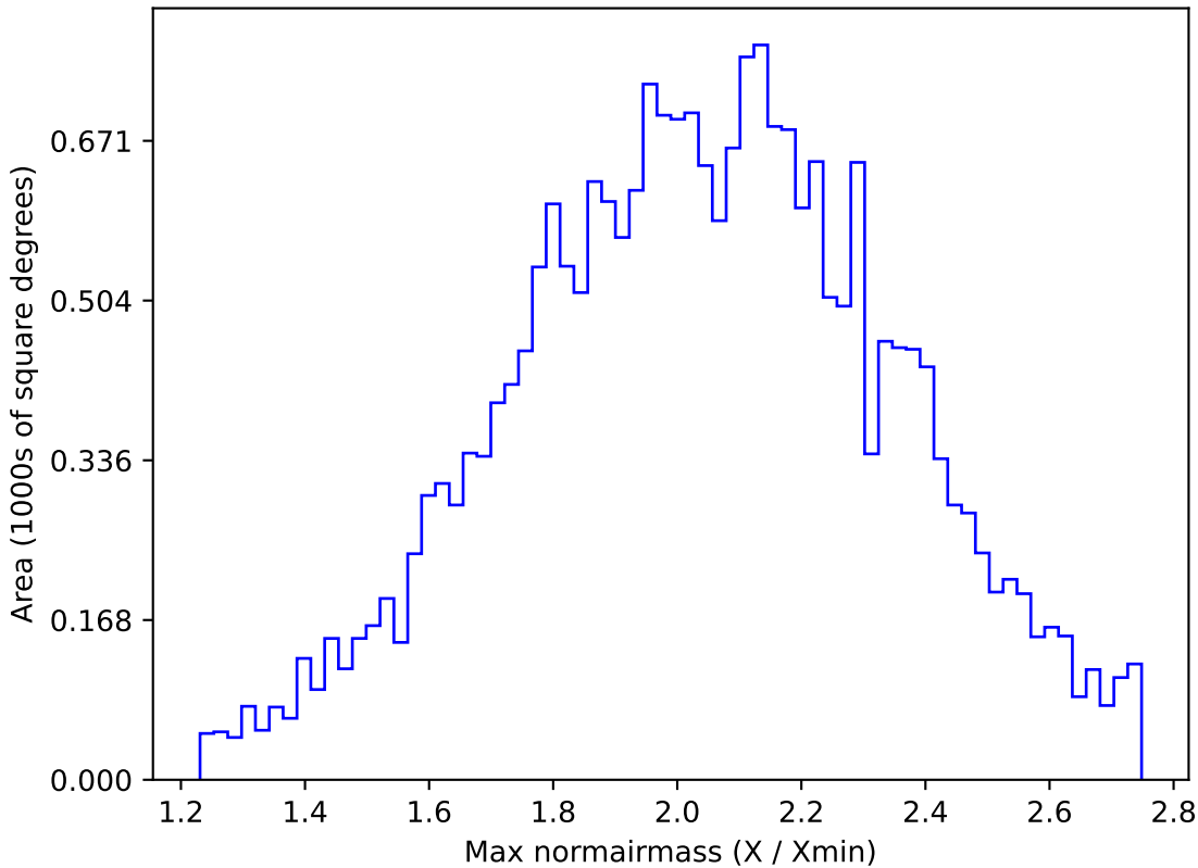
too_100_4v3.4_10yrs All sky y band: Max normairmass
