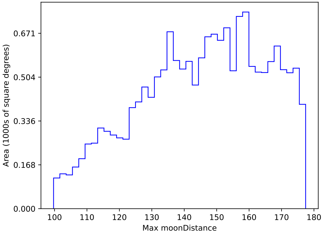
too_100_4v3.4_10yrs WFD y band: Max moonDistance
