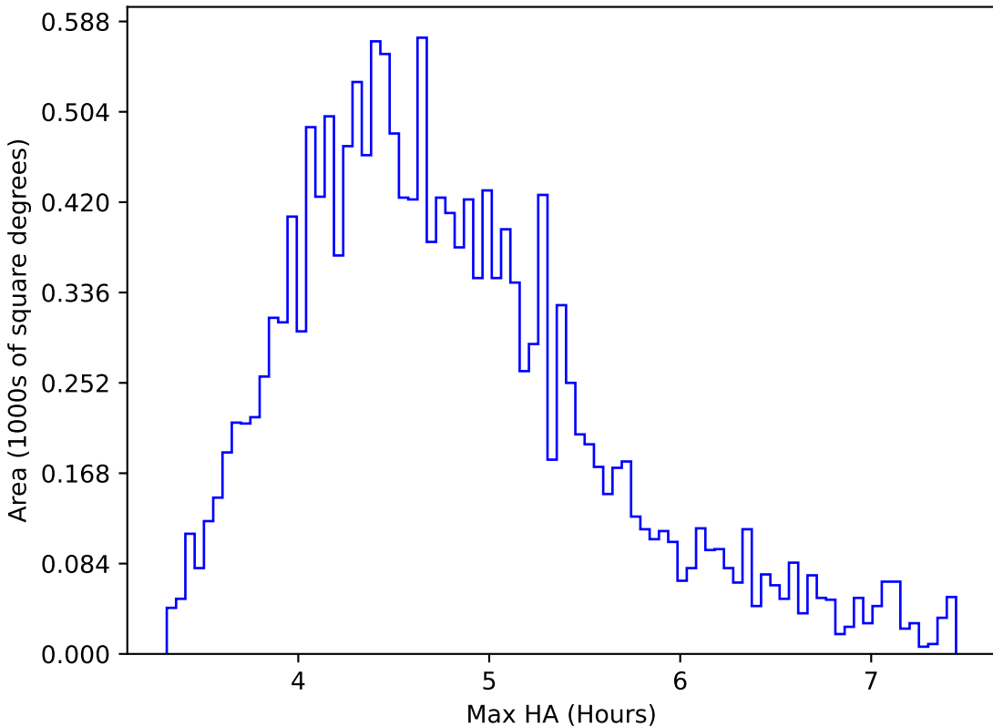
too_100_4v3.4_10yrs WFD y band: Max HA
