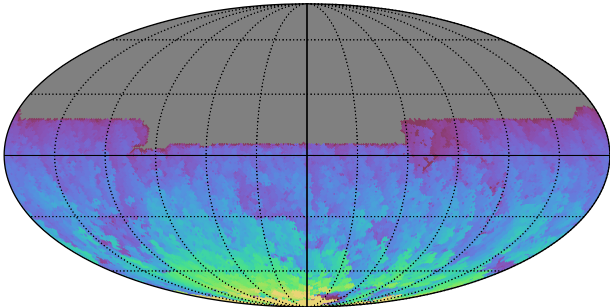
too_100_4v3.4_10yrs All sky y band: Max HA
