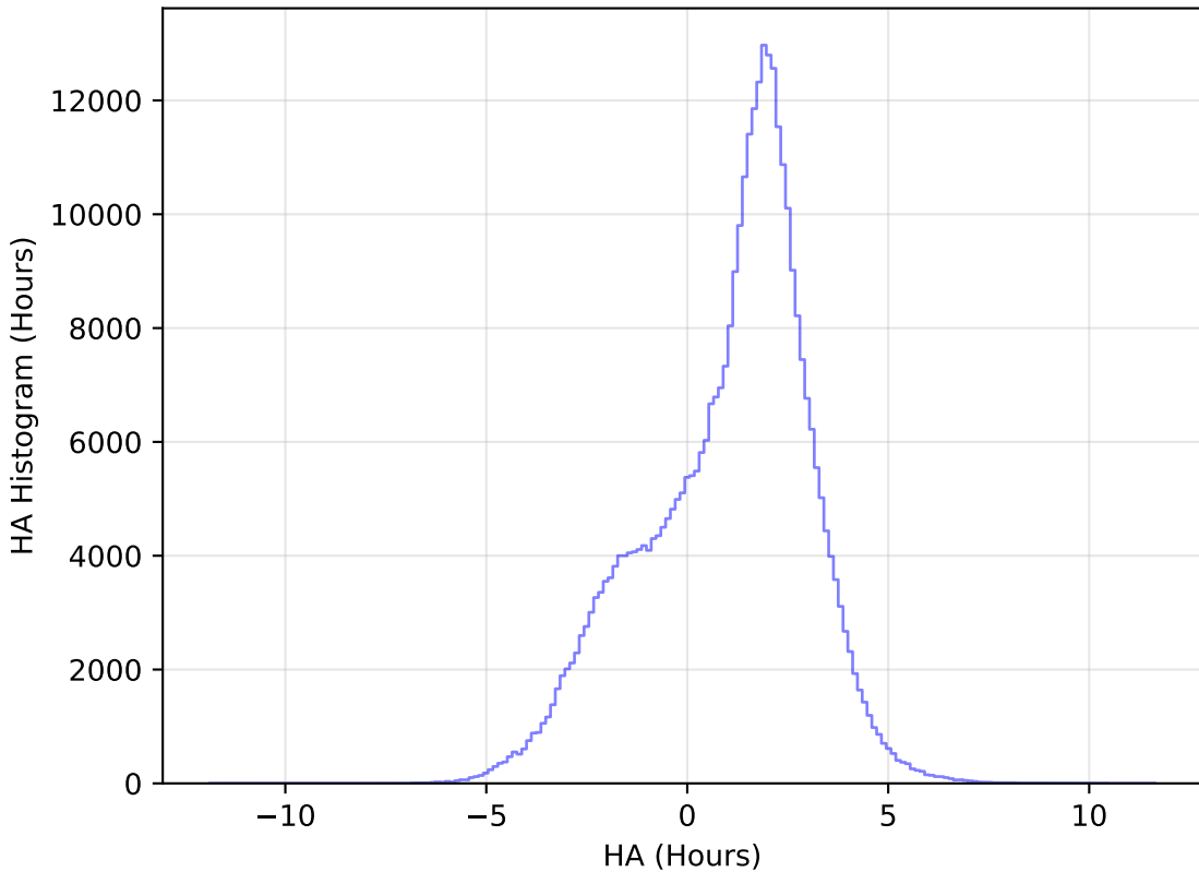
too_100_4v3.4_10yrs WFD y band: HA Histogram
