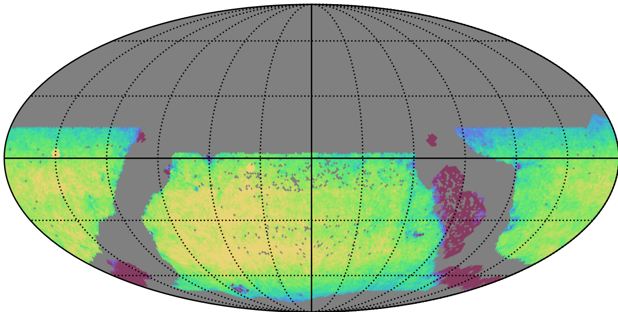
too_100_4v3.4_10yrs WFD y band: Exgal_CoaddM5
