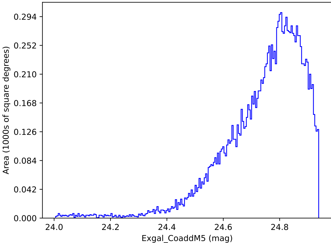
too_100_4v3.4_10yrs WFD y band: Exgal_CoaddM5
