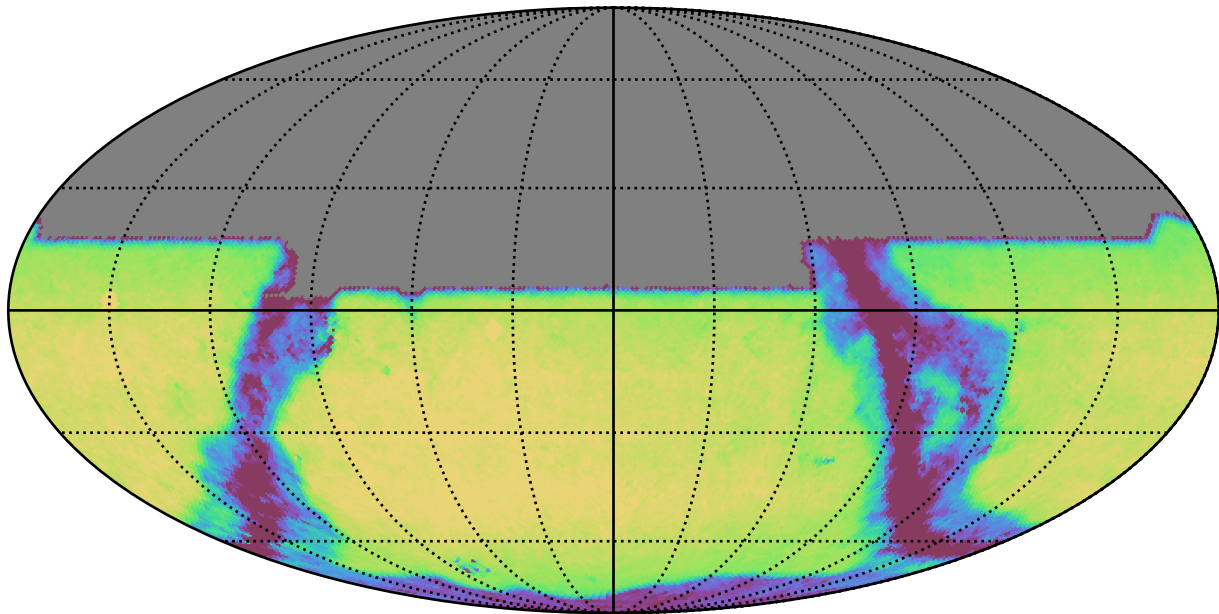
too_100_4v3.4_10yrs All sky y band: Exgal_CoaddM5
