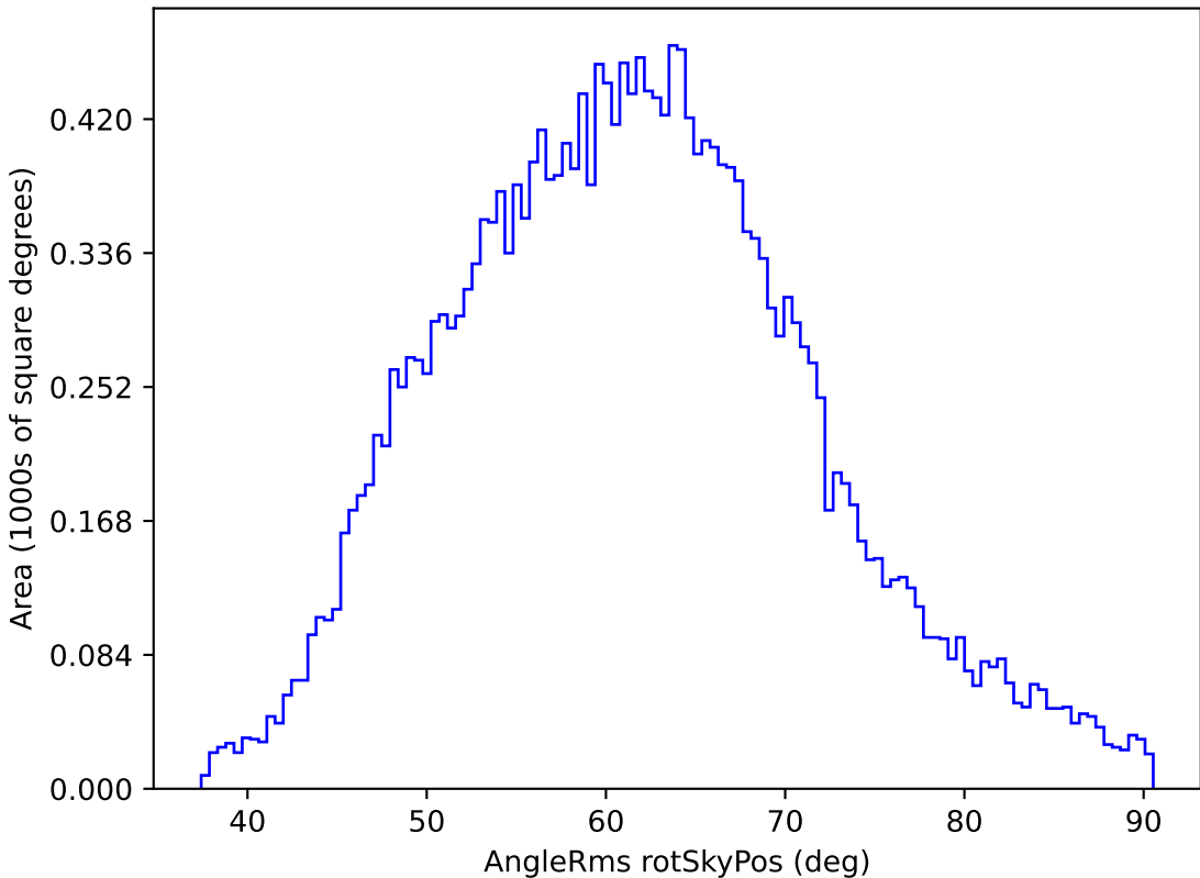
too_100_4v3.4_10yrs All sky y band: AngleRms rotSkyPos
