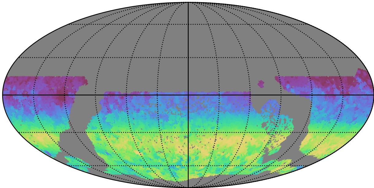
too_100_4v3.4_10yrs WFD z band: AngleRange rotSkyPos
