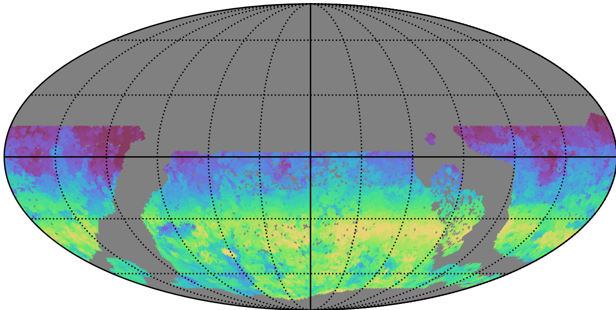
too_100_4v3.4_10yrs WFD y band: AngleRange rotSkyPos
