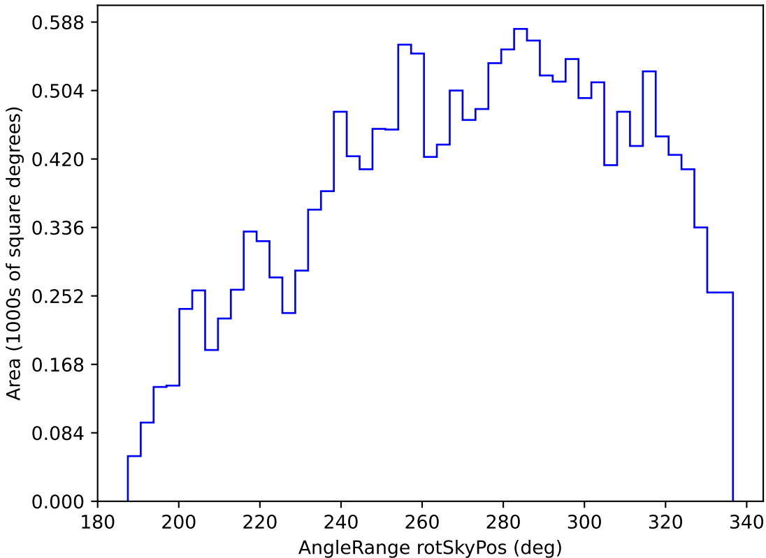
too_100_4v3.4_10yrs WFD y band: AngleRange rotSkyPos
