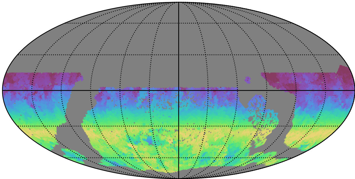
too_100_4v3.4_10yrs WFD r band: AngleRange rotSkyPos
