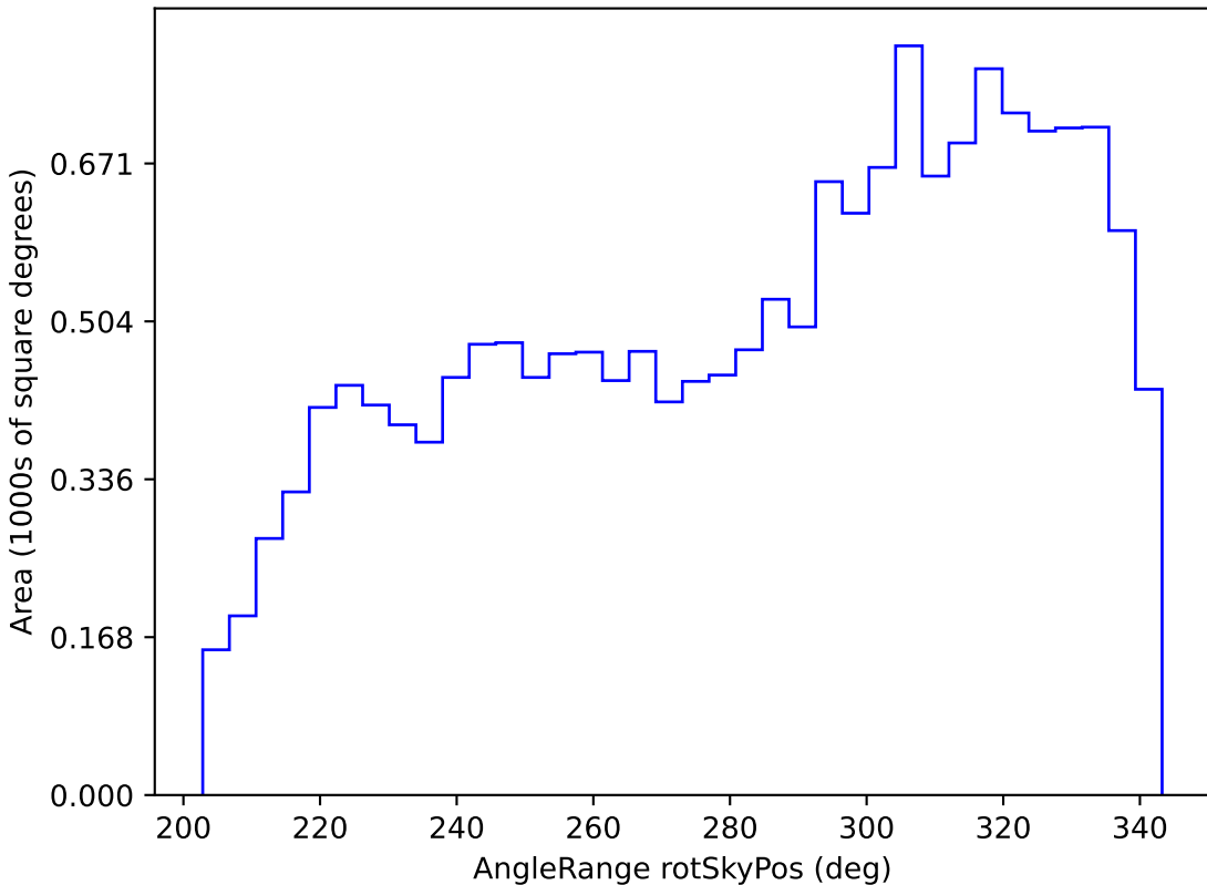
too_100_4v3.4_10yrs WFD r band: AngleRange rotSkyPos
