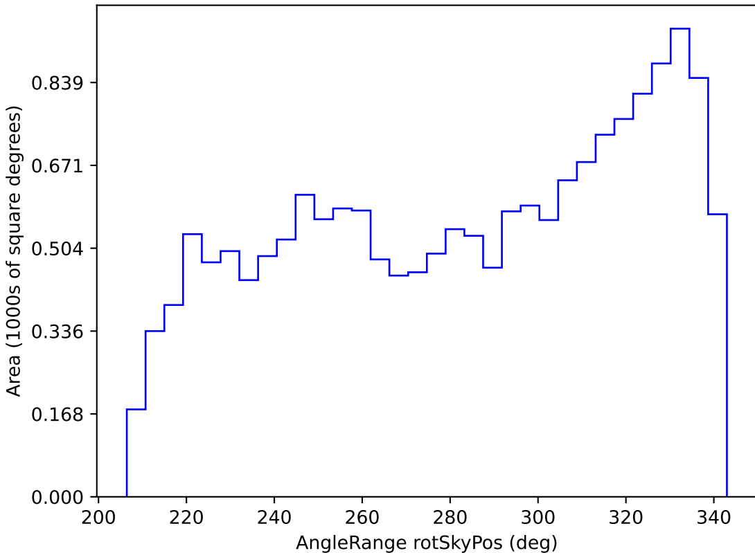
too_100_4v3.4_10yrs WFD i band: AngleRange rotSkyPos
