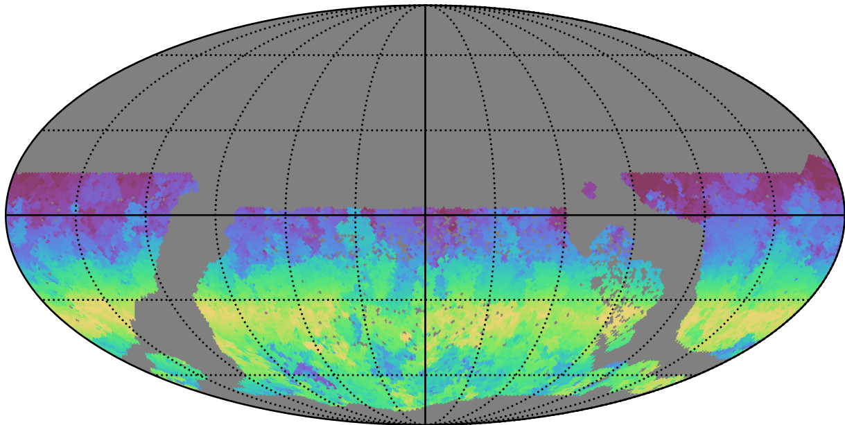
too_100_4v3.4_10yrs WFD g band: AngleRange rotSkyPos
