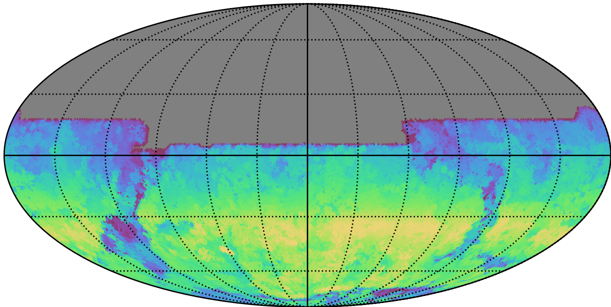
too_100_4v3.4_10yrs All sky y band: AngleRange rotSkyPos
