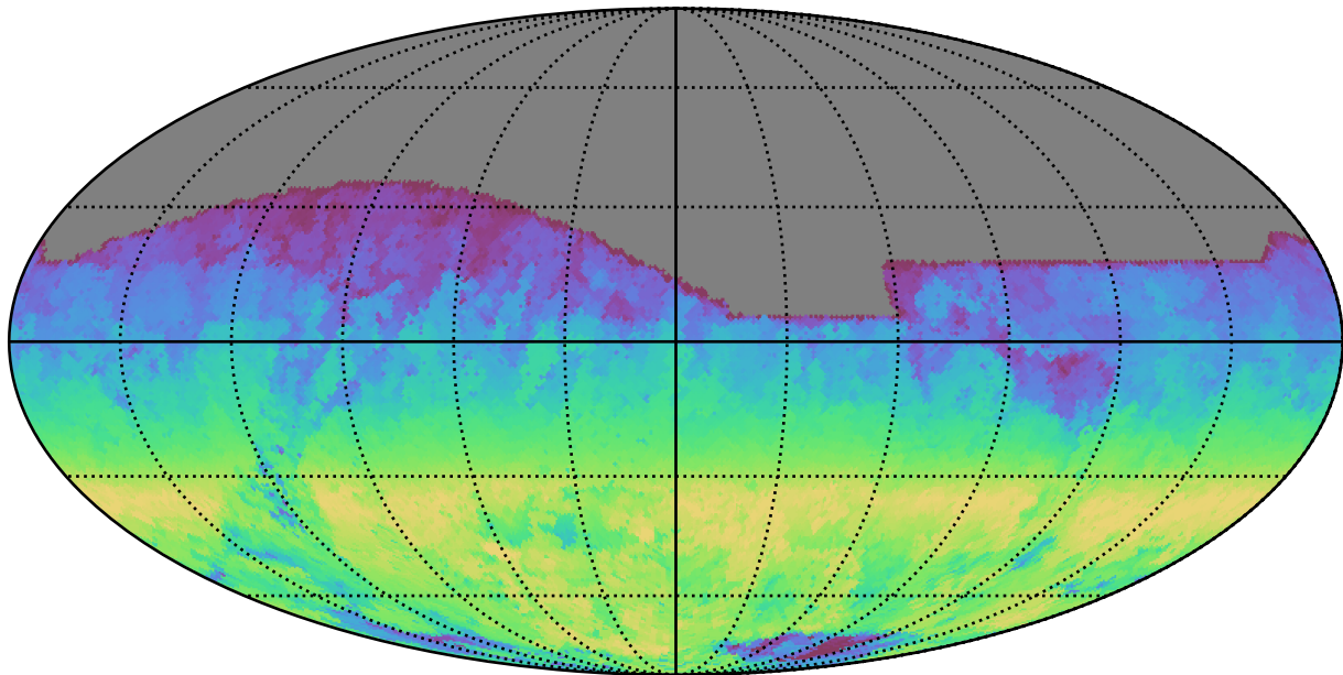
too_100_4v3.4_10yrs All sky r band: AngleRange rotSkyPos
