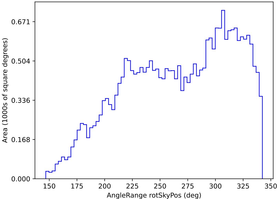
too_100_4v3.4_10yrs All sky r band: AngleRange rotSkyPos
