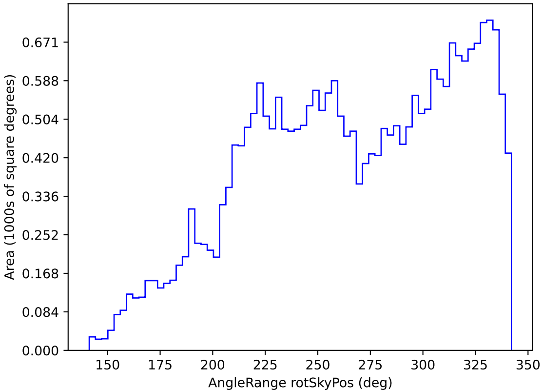
too_100_4v3.4_10yrs All sky i band: AngleRange rotSkyPos
