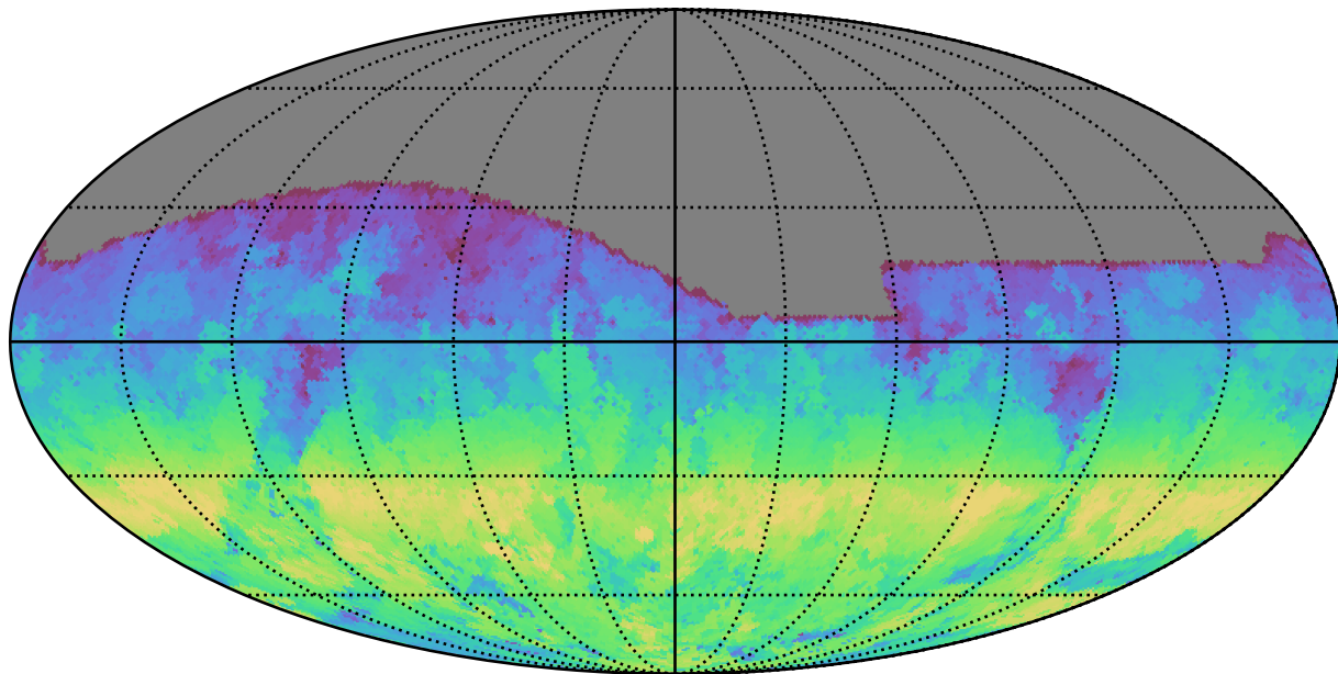
too_100_4v3.4_10yrs All sky g band: AngleRange rotSkyPos
