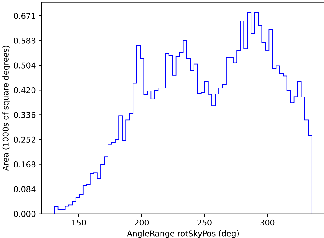
too_100_4v3.4_10yrs All sky g band: AngleRange rotSkyPos
