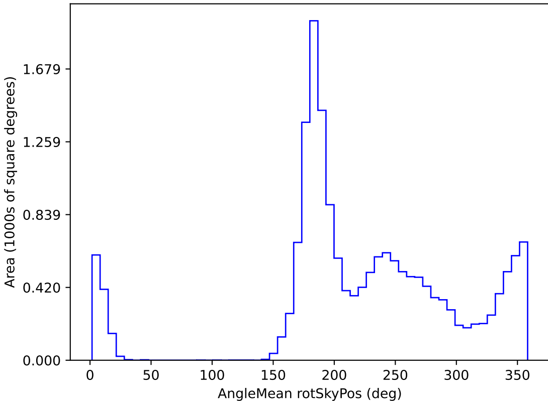
too_100_4v3.4_10yrs WFD y band: AngleMean rotSkyPos
