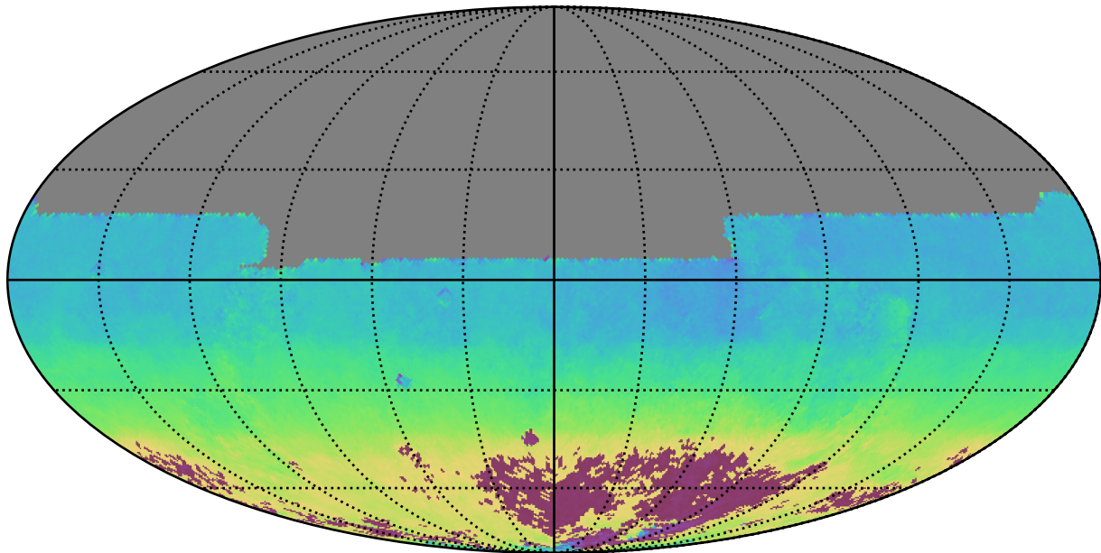
too_100_4v3.4_10yrs All sky y band: AngleMean rotSkyPos
