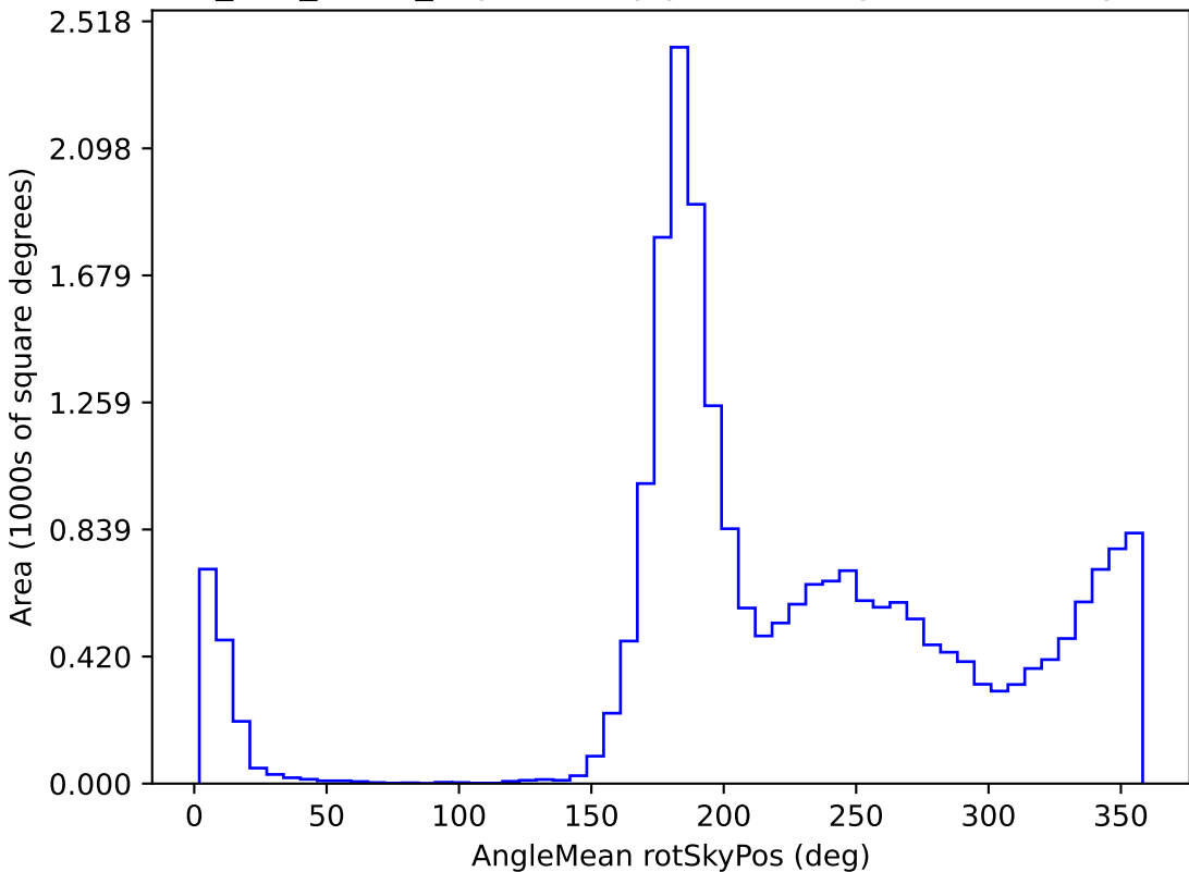
too_100_4v3.4_10yrs All sky y band: AngleMean rotSkyPos
