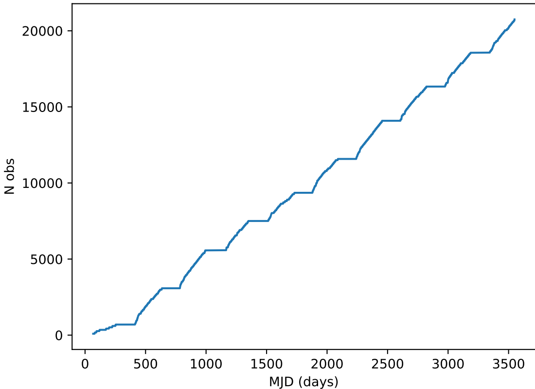
too_100_4v3.4_10yrs all bands: DD:ELAISS1 Cumulative NVisits
