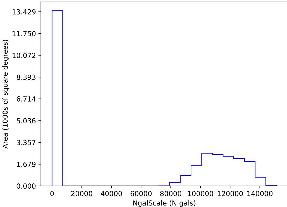
too_100_1v3.4_10yrs i: NgalScale
