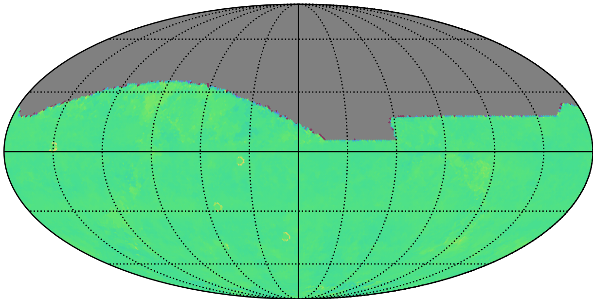
too_100_1v3.4_10yrs z: Kuiper rotTelPos
