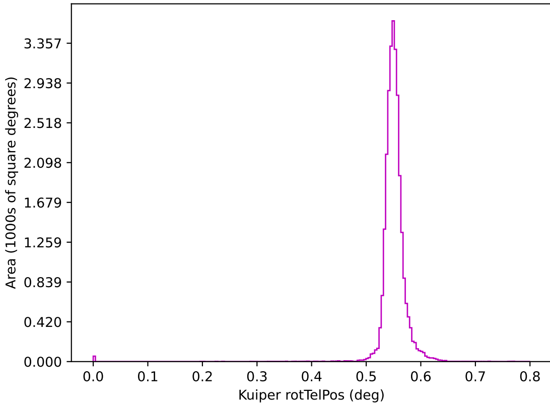
too_100_1v3.4_10yrs z: Kuiper rotTelPos
