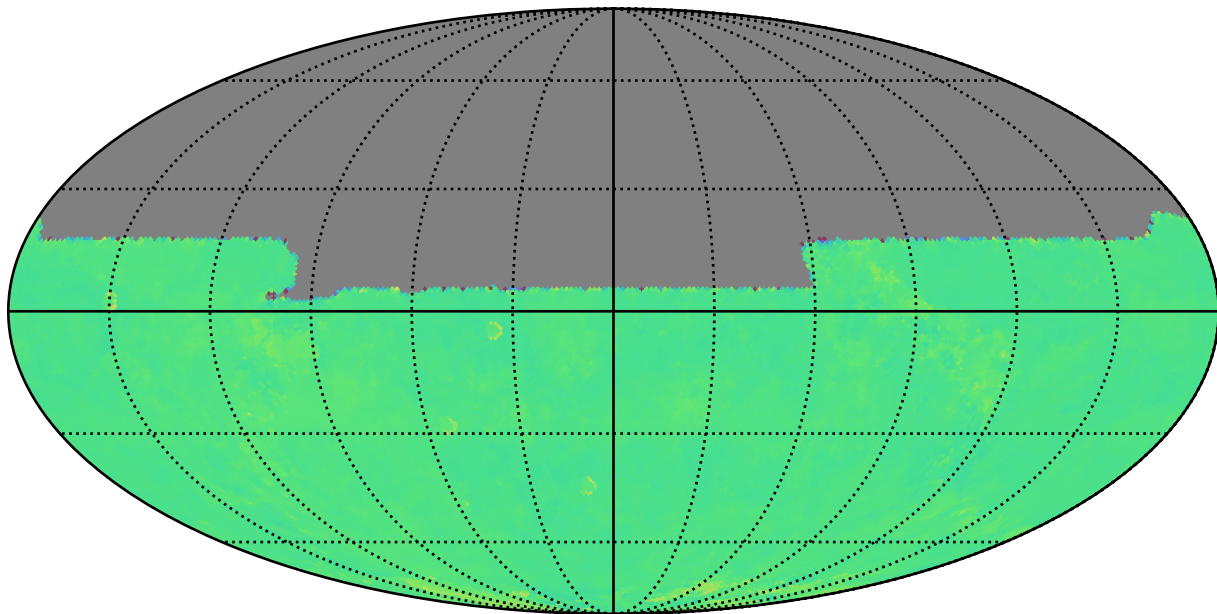
too_100_1v3.4_10yrs y: Kuiper rotTelPos
