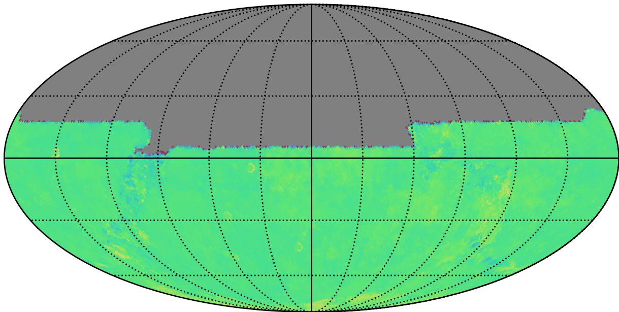
too_100_1v3.4_10yrs u: Kuiper rotTelPos
