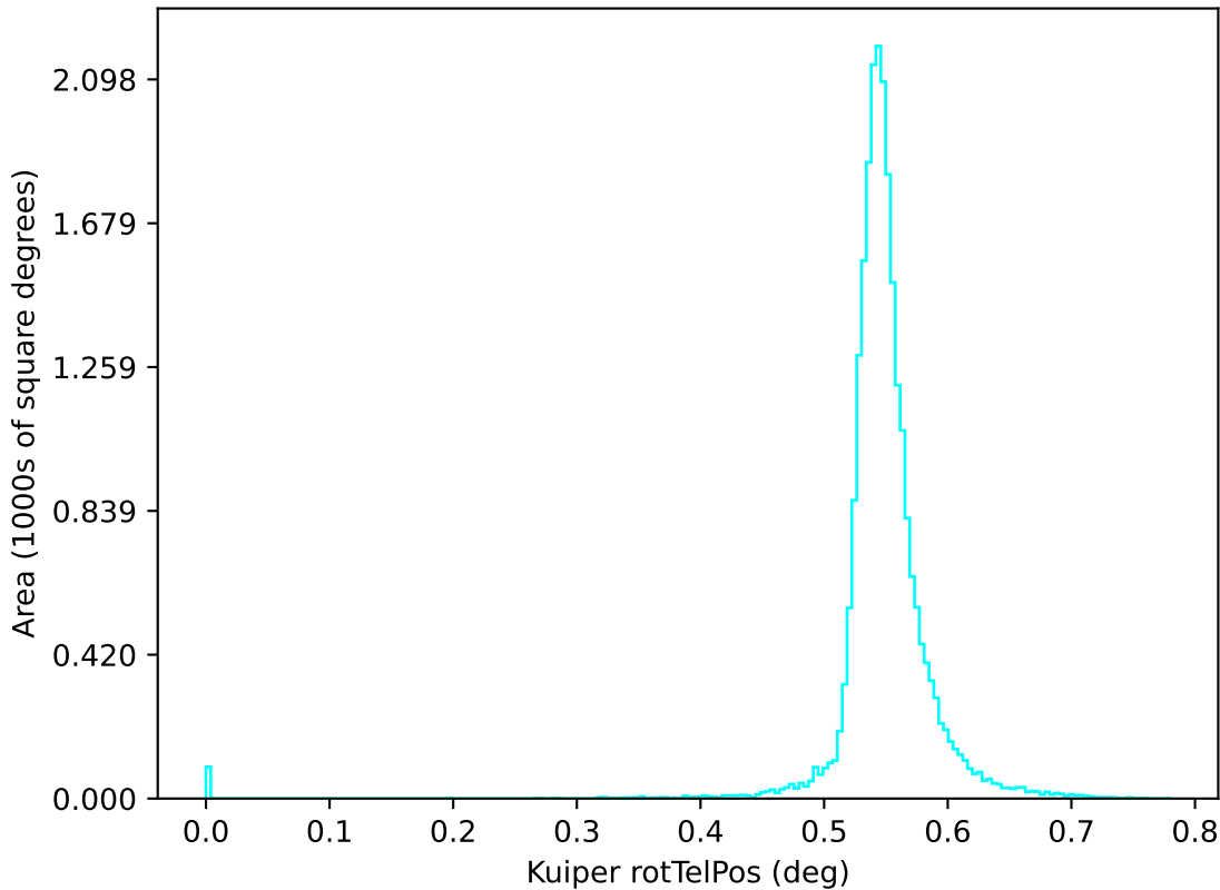
too_100_1v3.4_10yrs u: Kuiper rotTelPos
