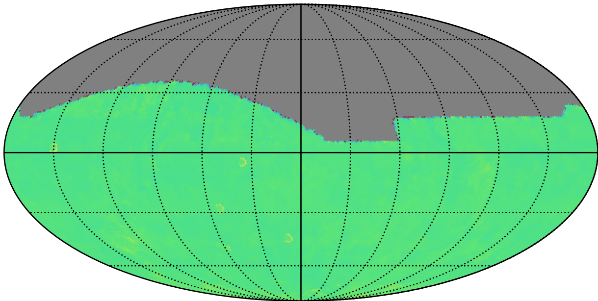
too_100_1v3.4_10yrs r: Kuiper rotTelPos
