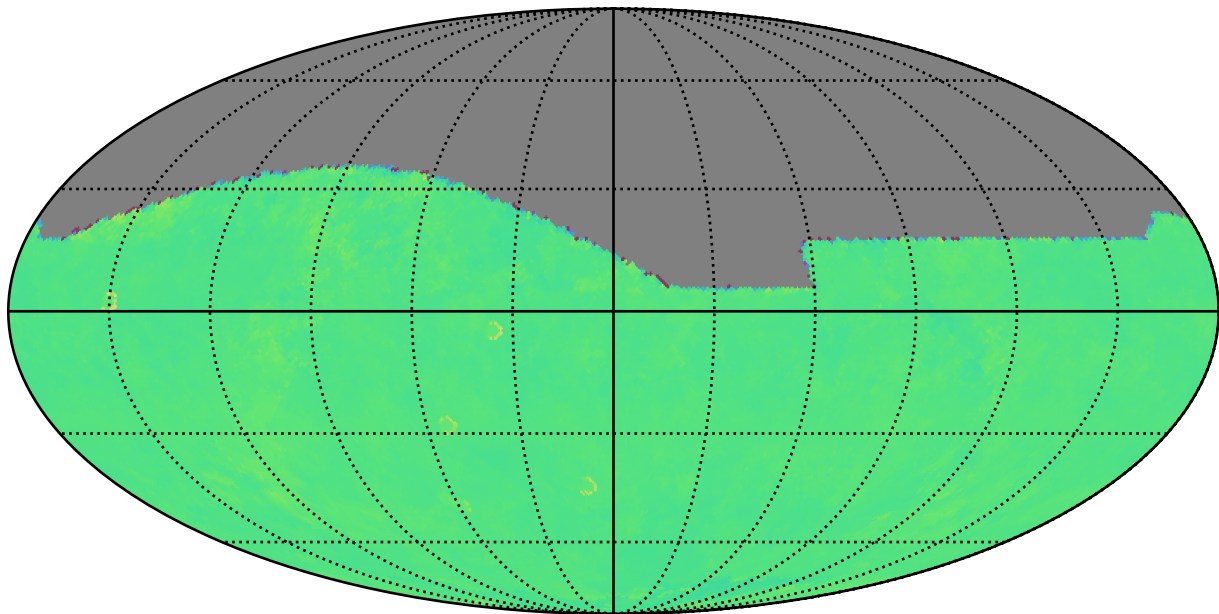
too_100_1v3.4_10yrs i: Kuiper rotTelPos
