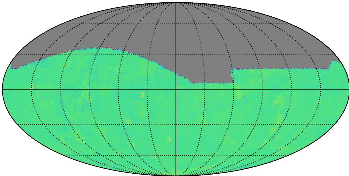
too_100_1v3.4_10yrs g: Kuiper rotTelPos
