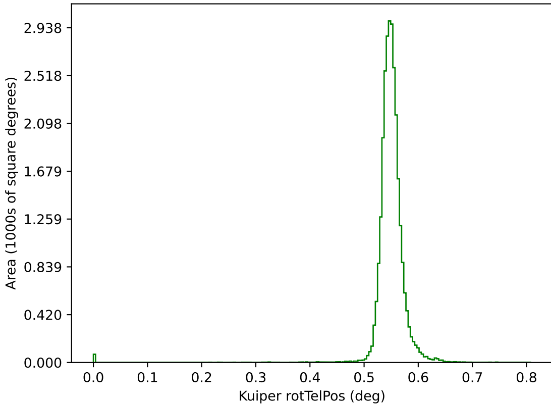
too_100_1v3.4_10yrs g: Kuiper rotTelPos
