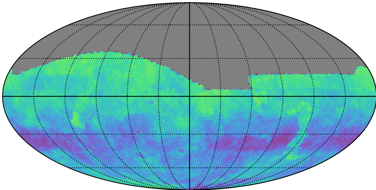
too_100_1v3.4_10yrs g: Kuiper rotSkyPos
