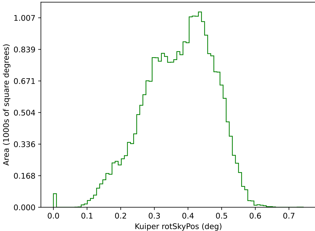
too_100_1v3.4_10yrs g: Kuiper rotSkyPos
