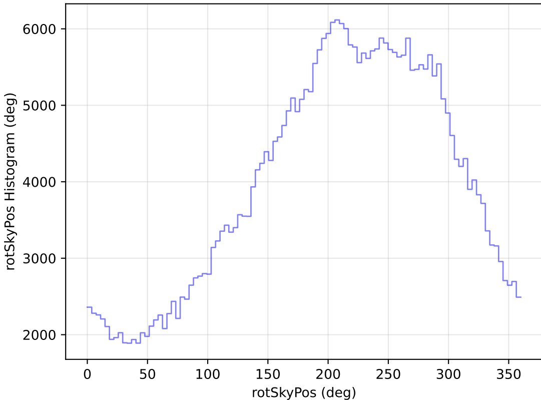
too_100_1v3.4_10yrs WFD y band: rotSkyPos Histogram
