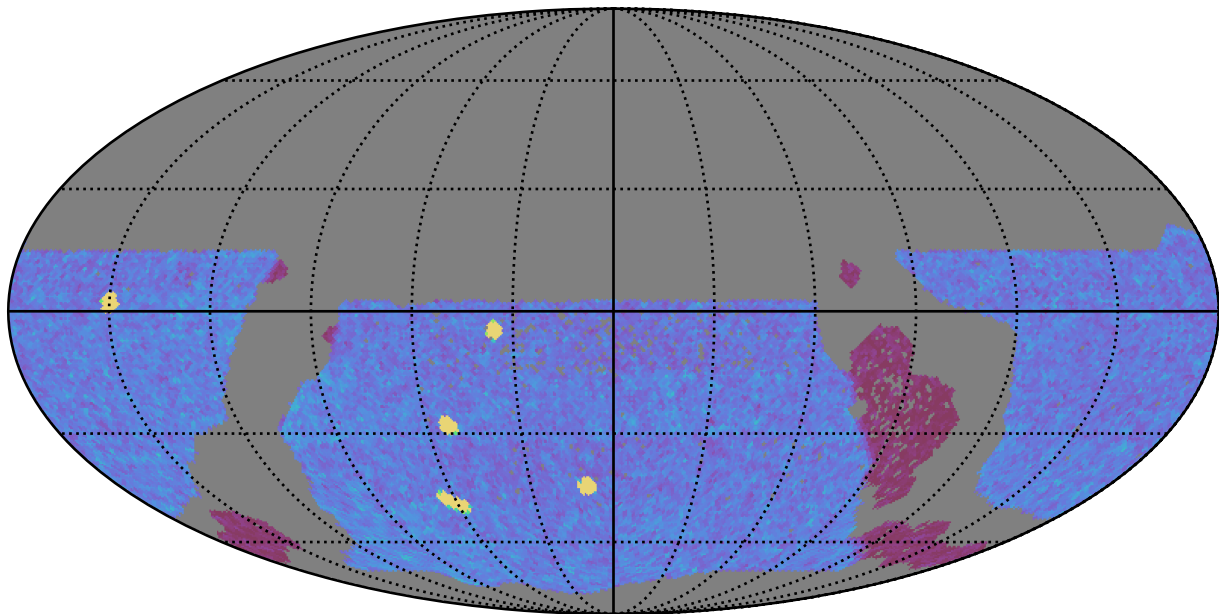
too_100_1v3.4_10yrs WFD y band: NVisits
