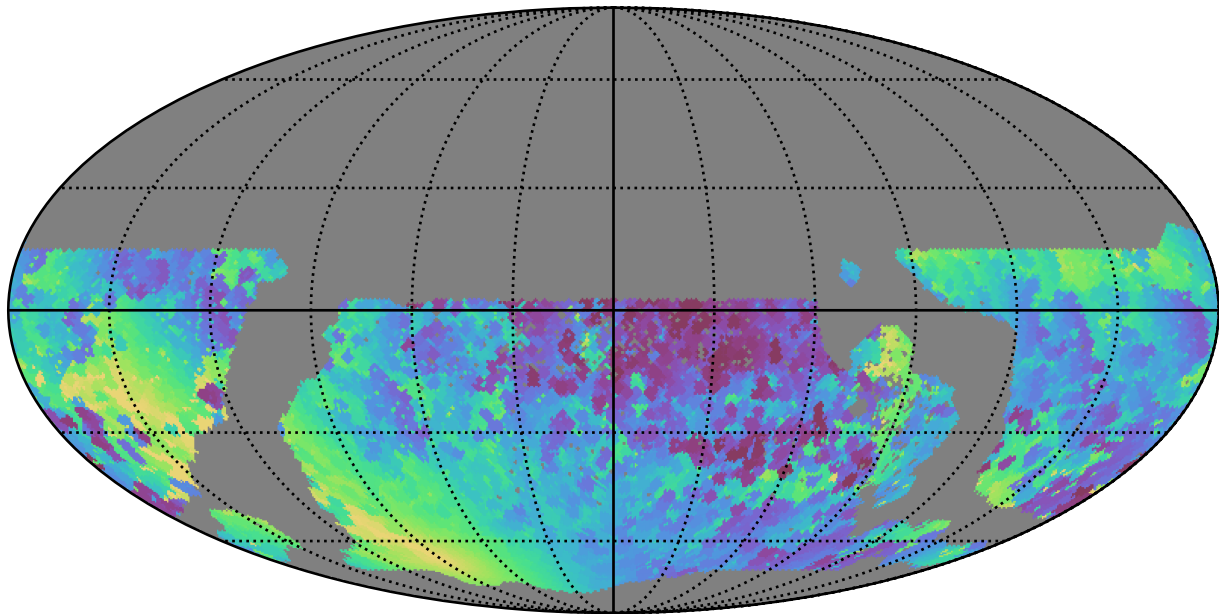
too_100_1v3.4_10yrs WFD y band: Min solarElong
