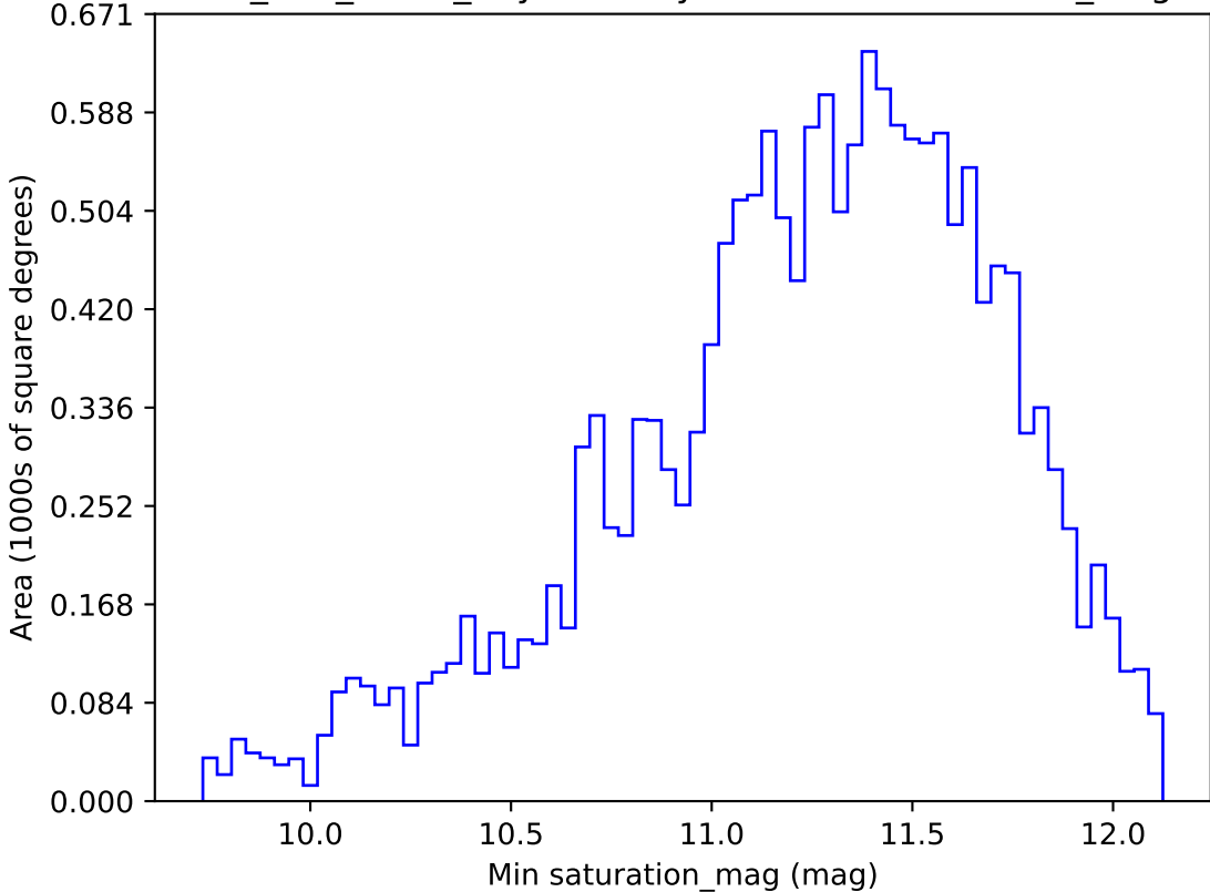
too_100_1v3.4_10yrs WFD y band: Min saturation_mag
